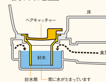
●排水トラップ断面図
